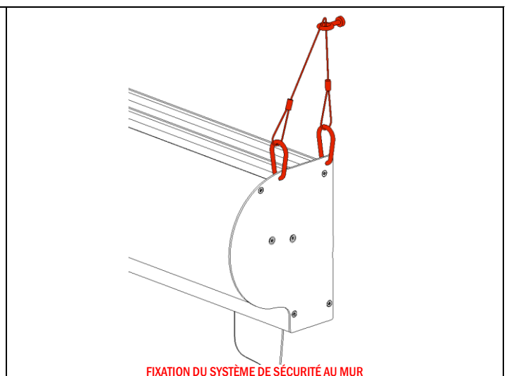
FIXATION DU SYSTÈME DE SÉCURITÉ AU MUR
